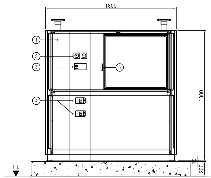
정면도
