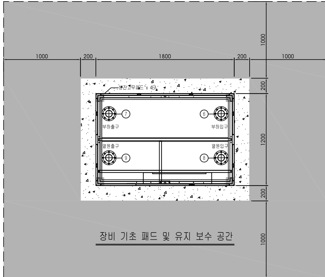
평면도
