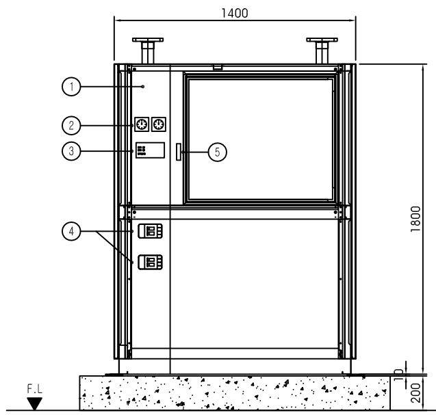
정면도
