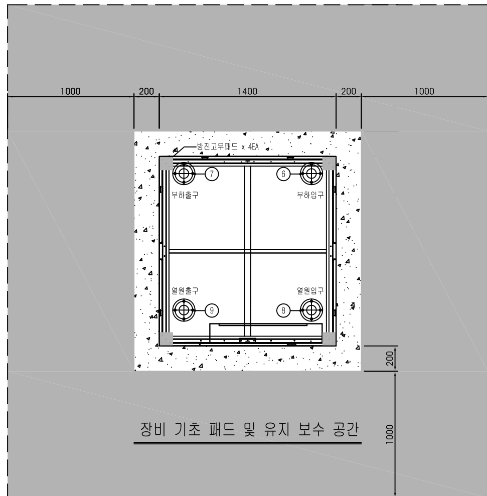
평면도
