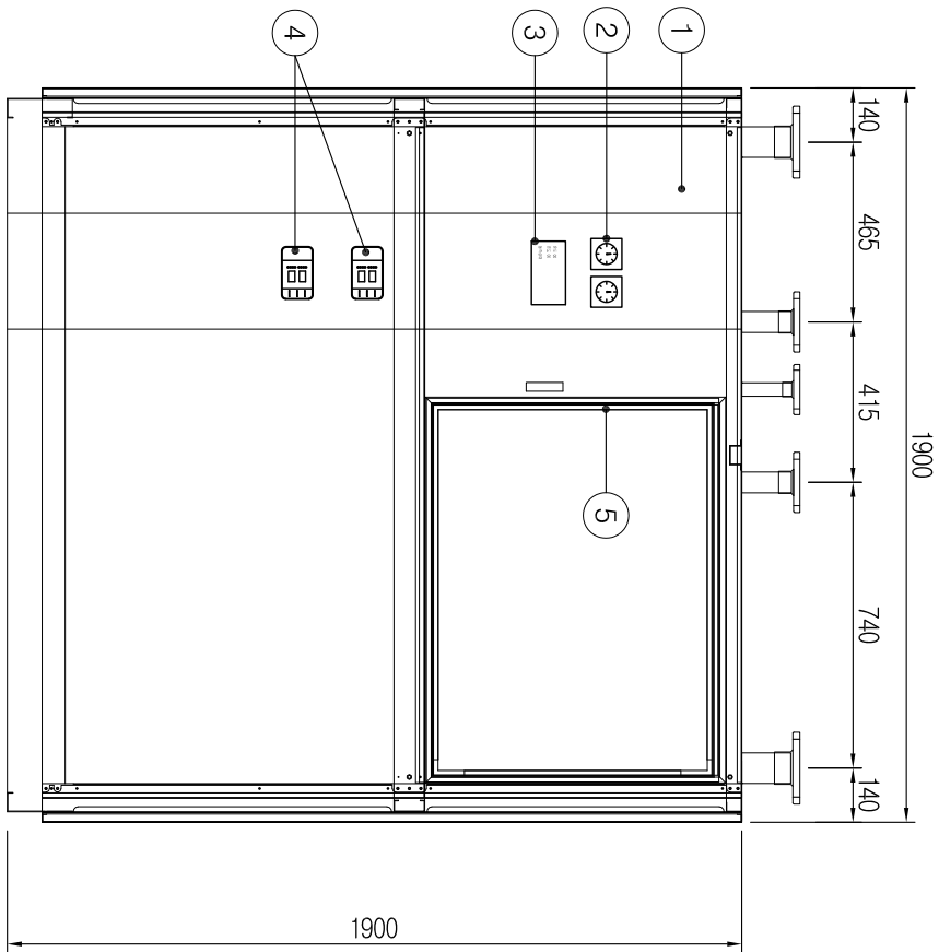
정면도
