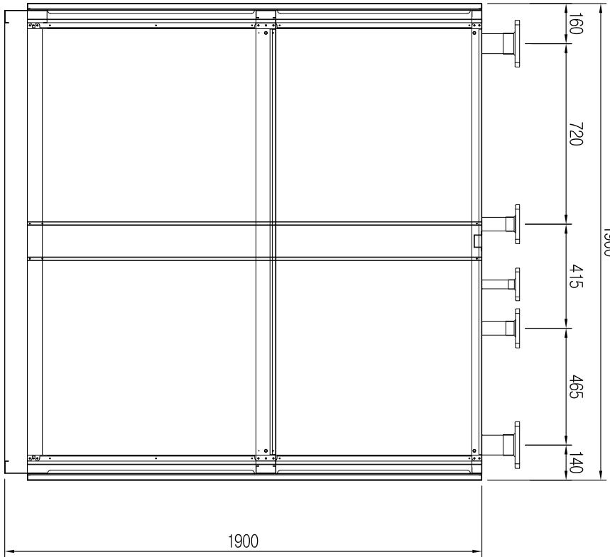
배면도
