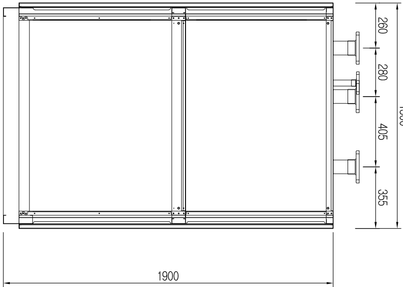
측면도
