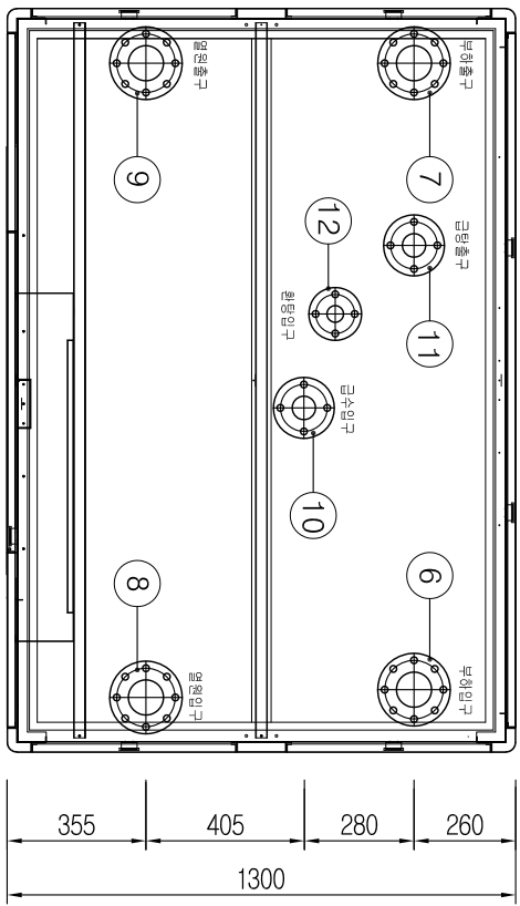
평면도
