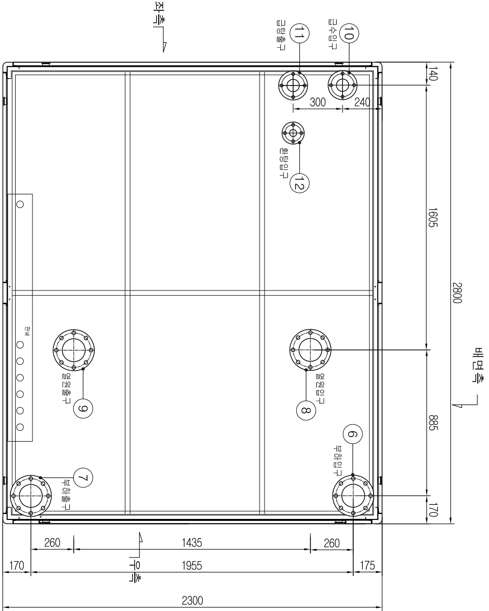
평면도
