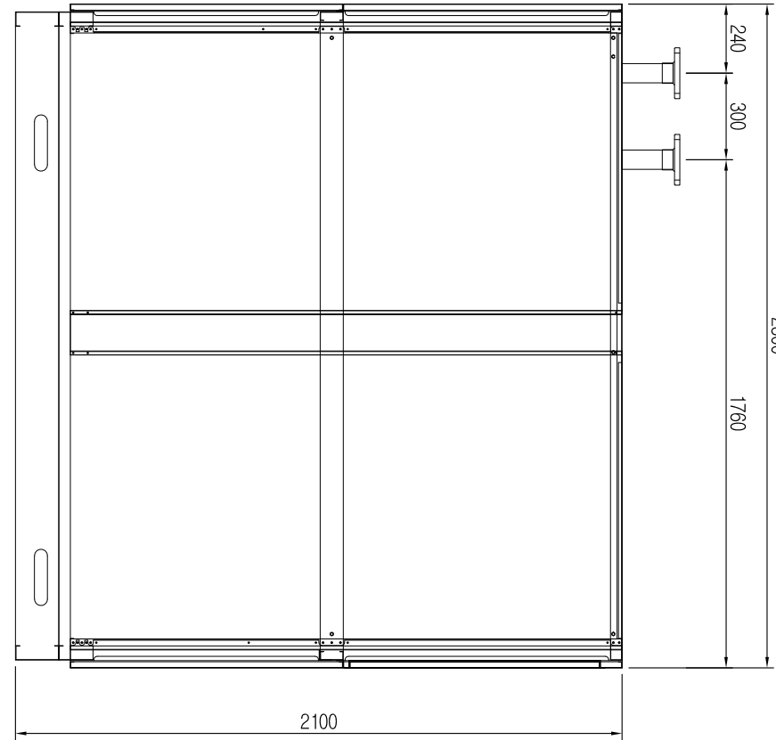
좌측면도
