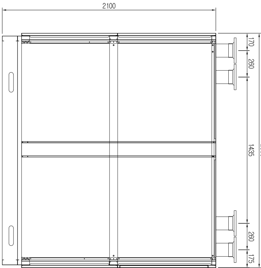
우측면도
