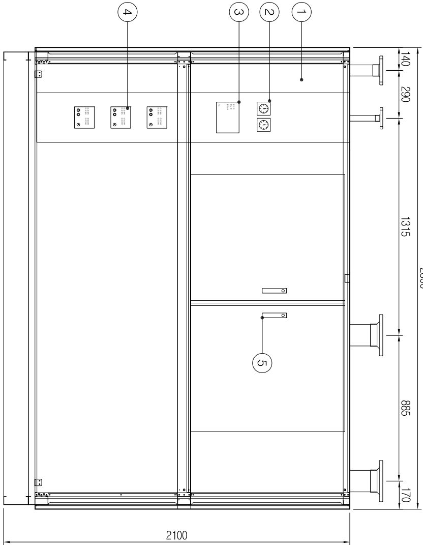
정면도(모니터측)
