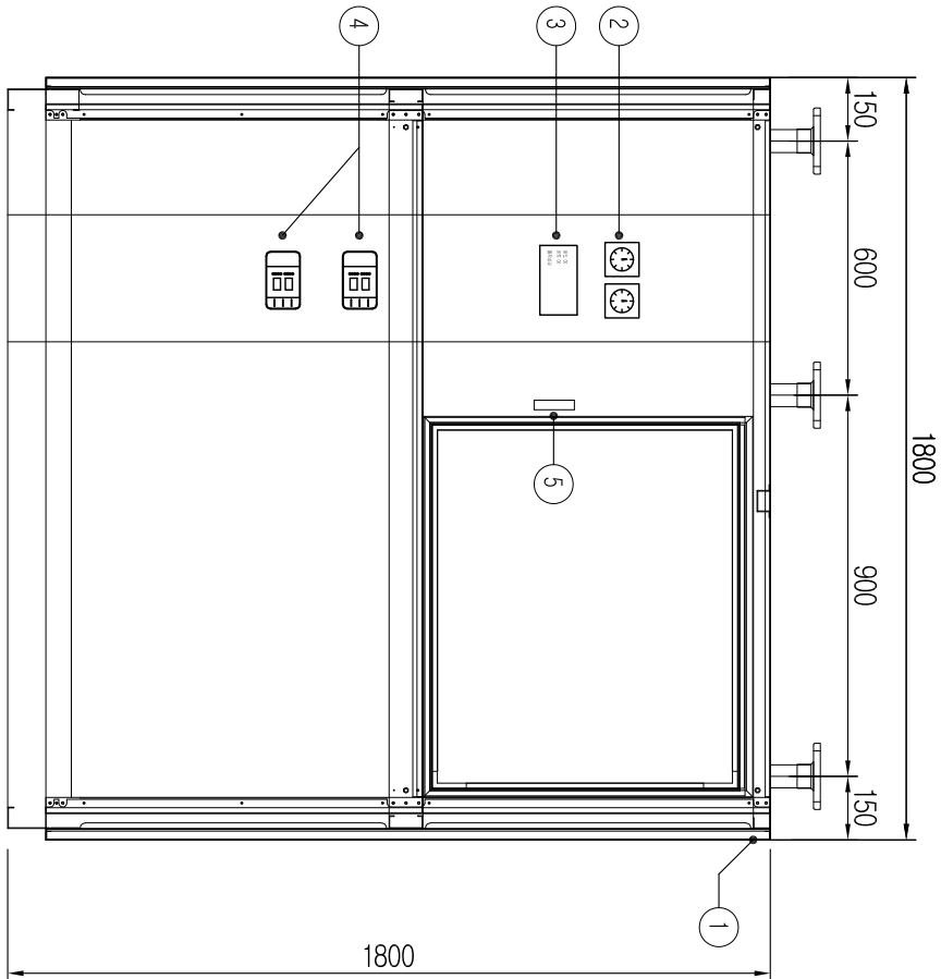
정면도
