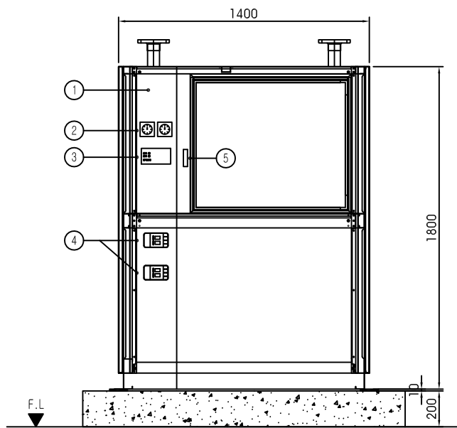
정면도
