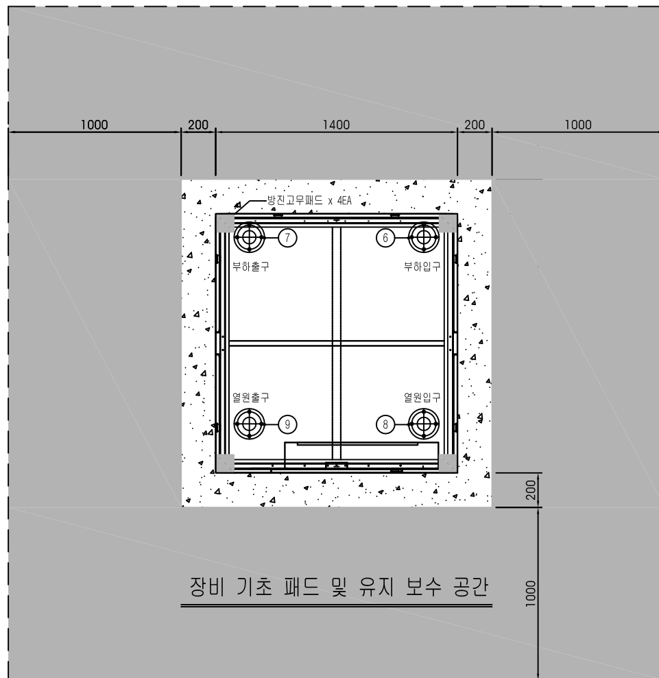
평면도
